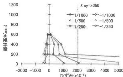
図 11 曲げ補強鉄筋ひずみ(No.3)
