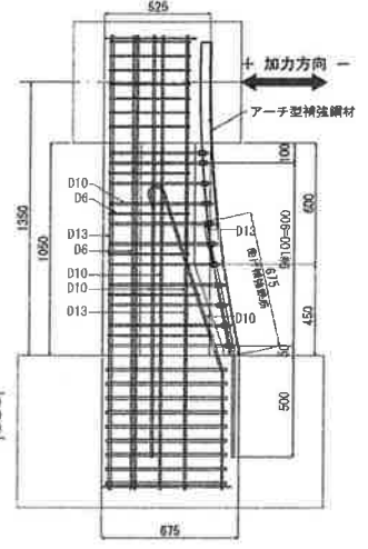
(No.2試験体) 図3 試験体側面図
