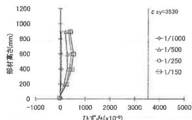
図 14 鋼板ひずみ(No.3)
