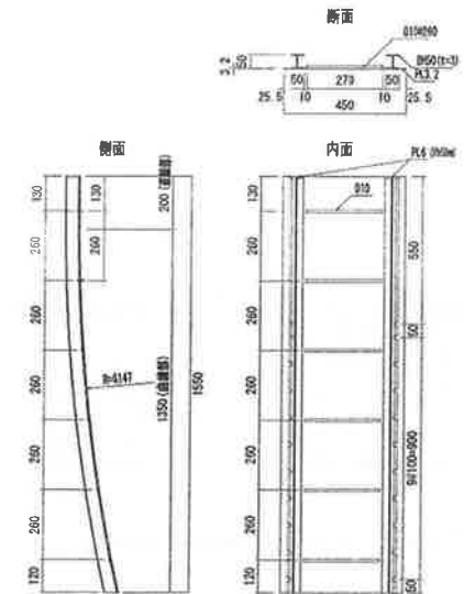
図4 アーチ型補強鋼材 (No.2試験体)
